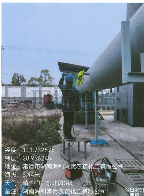
有组织废气采样
